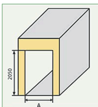
05 A = jmenovitá šířka dveří +(16 - 17 cm)
