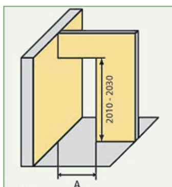
02 A = jmenovitá šířka dveří +(12 - 13 cm)
