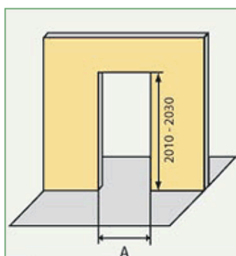
01 A = jmenovitá šířka dveří +(8 - 10 cm)
